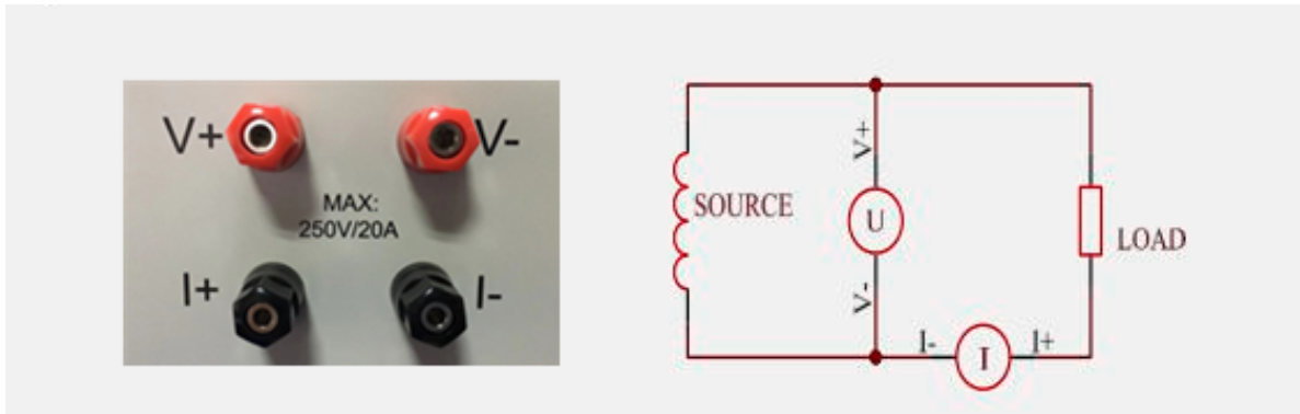
(图 6-1 电流表内接法--适用于小电流接法)
