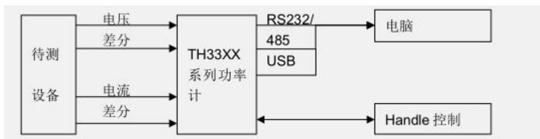
(图 7-1 系统构造)
