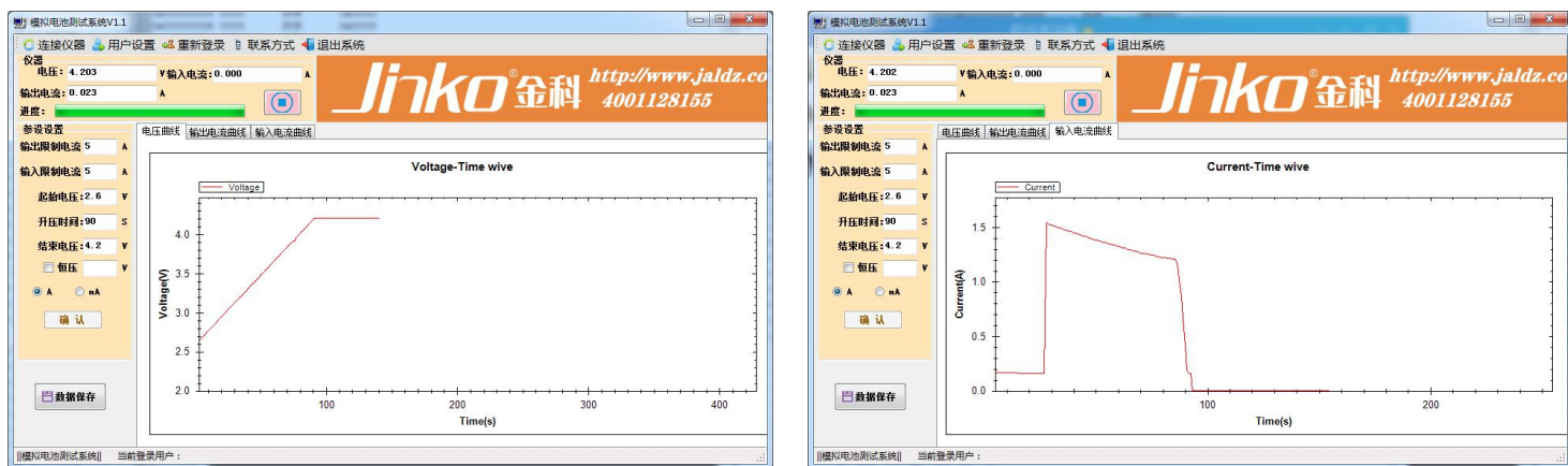
图5.3.1 – 1 充电曲线
