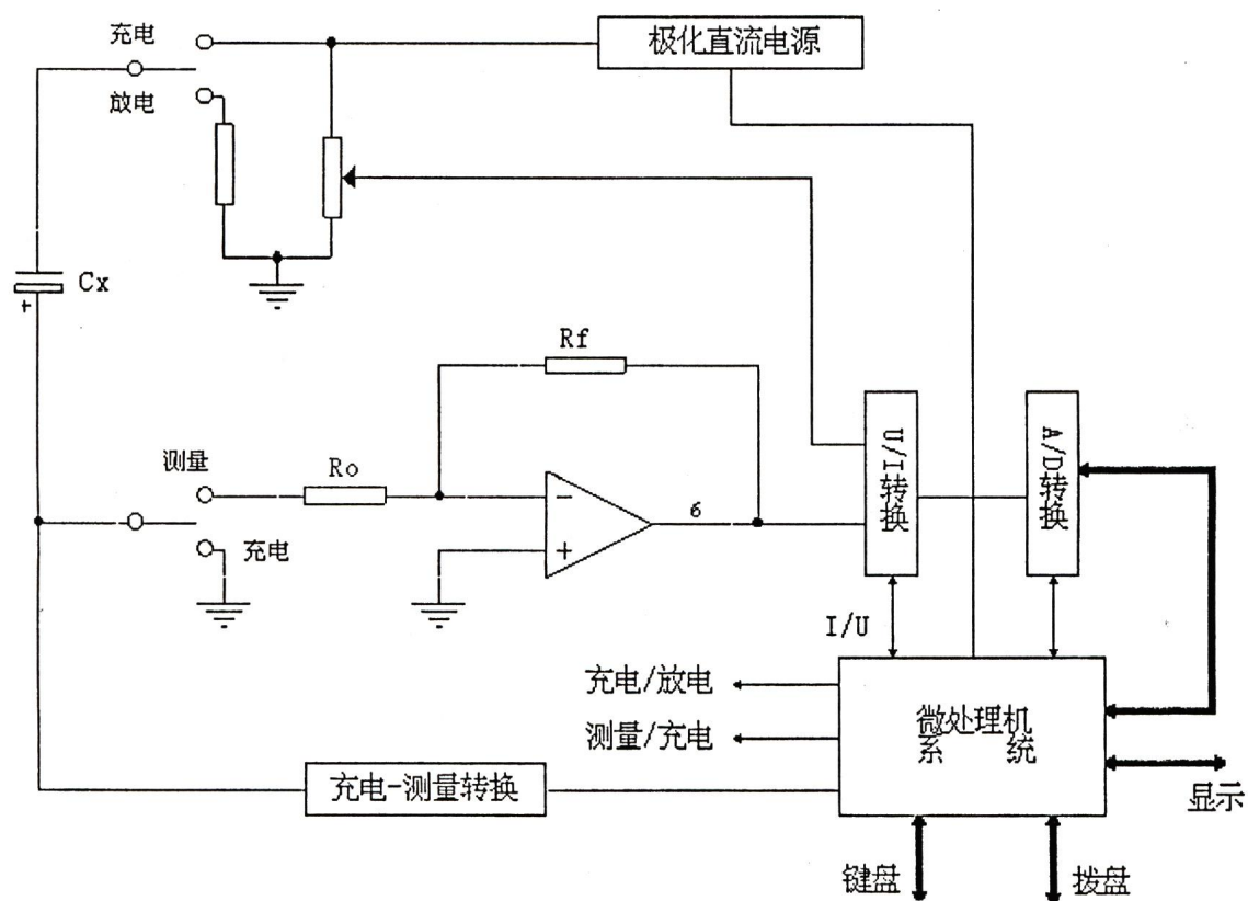
图 2 仪器框图
