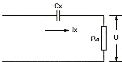
图 1 测量原理
